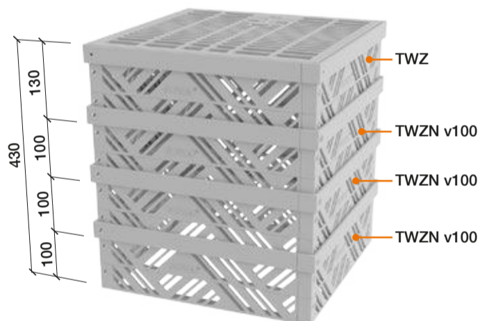
Komponenty šachty s perforovaným víkem výšky 430 mm
