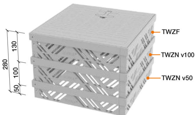
Komponenty šachty s neperforovaným víkem výšky 280 mm
